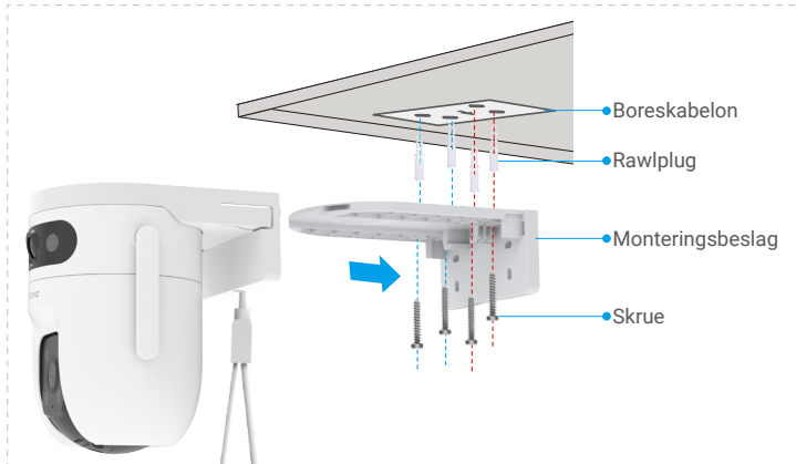
Fig. 1 Montering i loft
